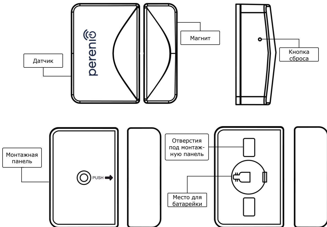
Рисунок 2: Составные части датчика открытия PECWS01
