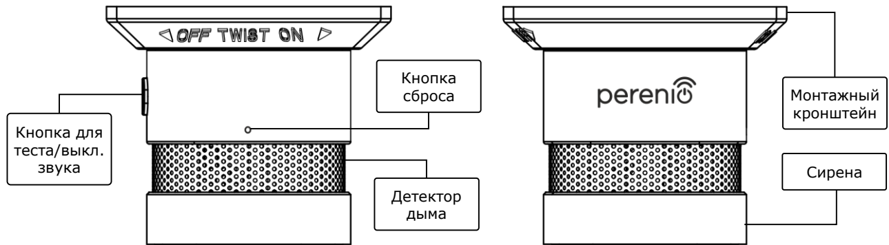
Рисунок 2: Кнопки и составные части датчика дыма PECSS01
