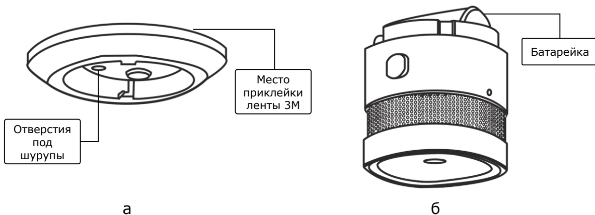
Рисунок 6: Крепление датчика дыма на дюбели или клейкую ленту 3М
