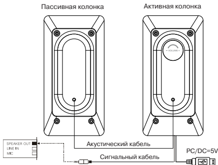
Рис. 2. Схема подключения
