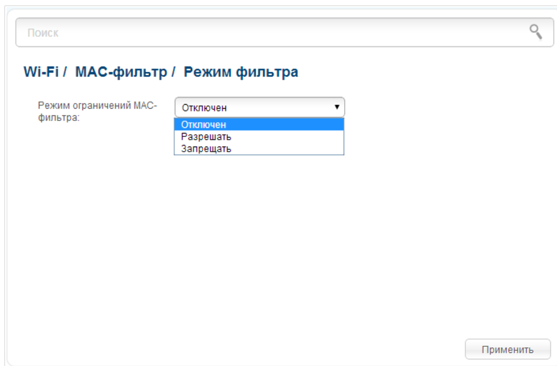
Рисунок 116. Страница для настройки MAC-фильтра для беспроводной сети.
