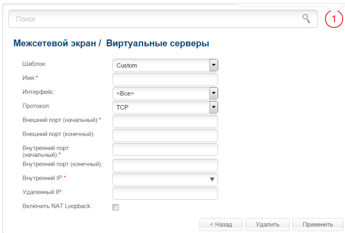
Рисунок 140. Страница добавления виртуального сервера.
