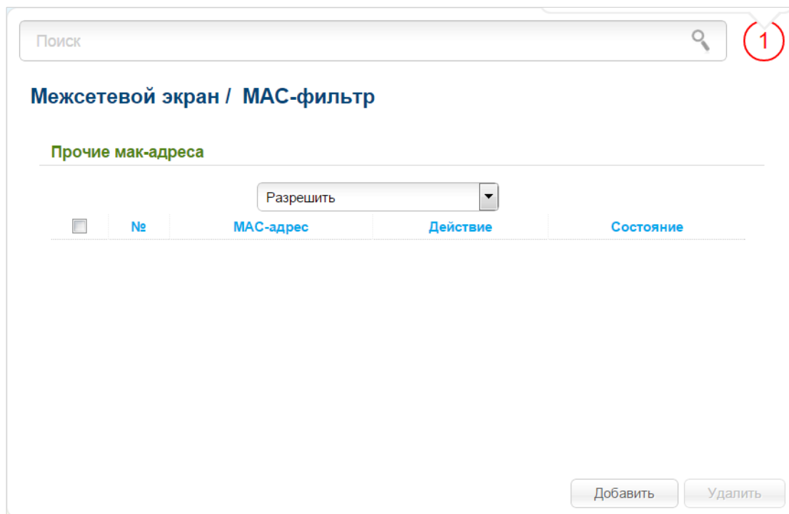
Рисунок 142. Страница Межсетевой экран / MAC-фильтр .
