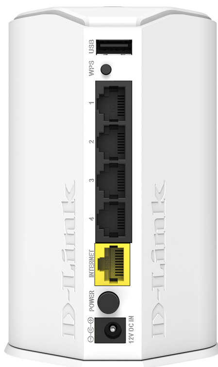
Рисунок 2. Вид задней панели DIR-620A.
