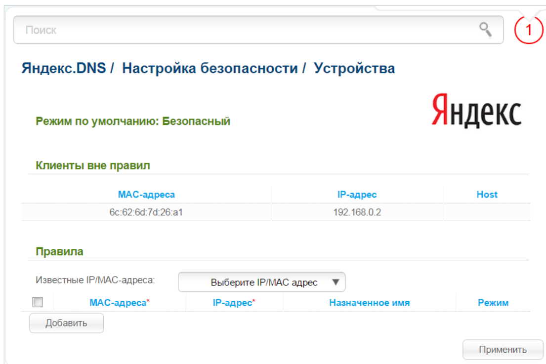
Рисунок 159. Страница Яндекс.DNS / Настройка безопасности / Устройства .
