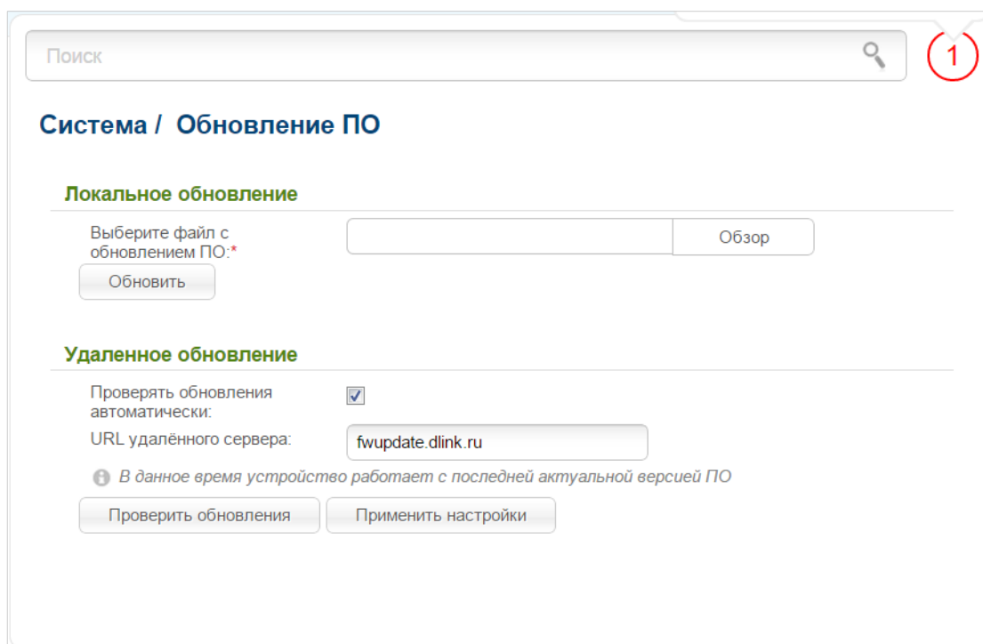
Рисунок 164. Страница Система / Обновление ПО .
