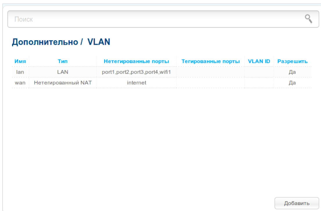
Рисунок 123. Страница Дополнительно / VLAN .
