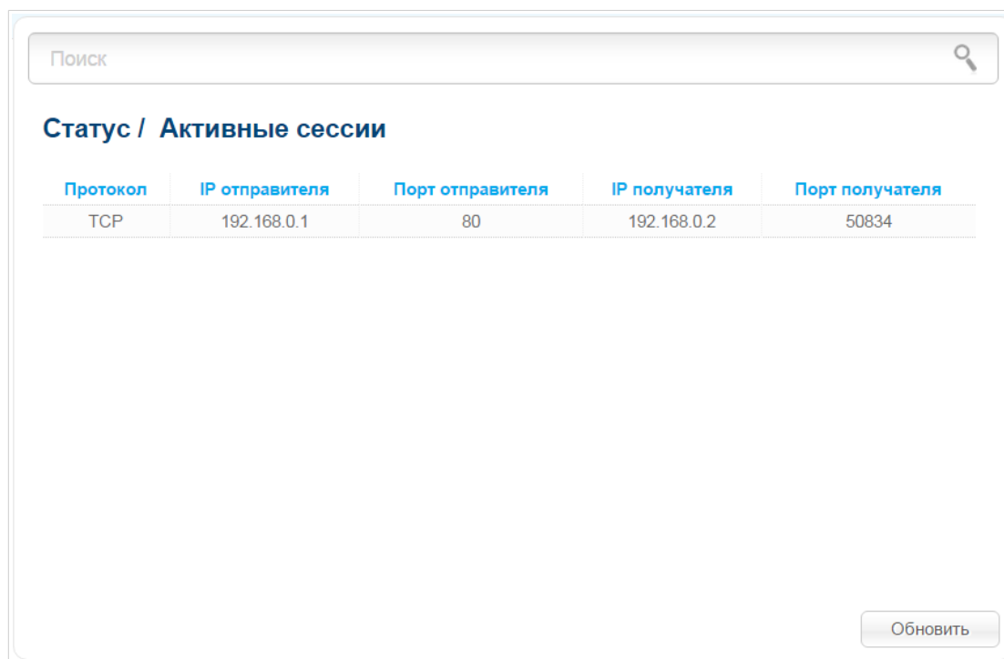
Рисунок 62. Страница Статус / Активные сессии .
