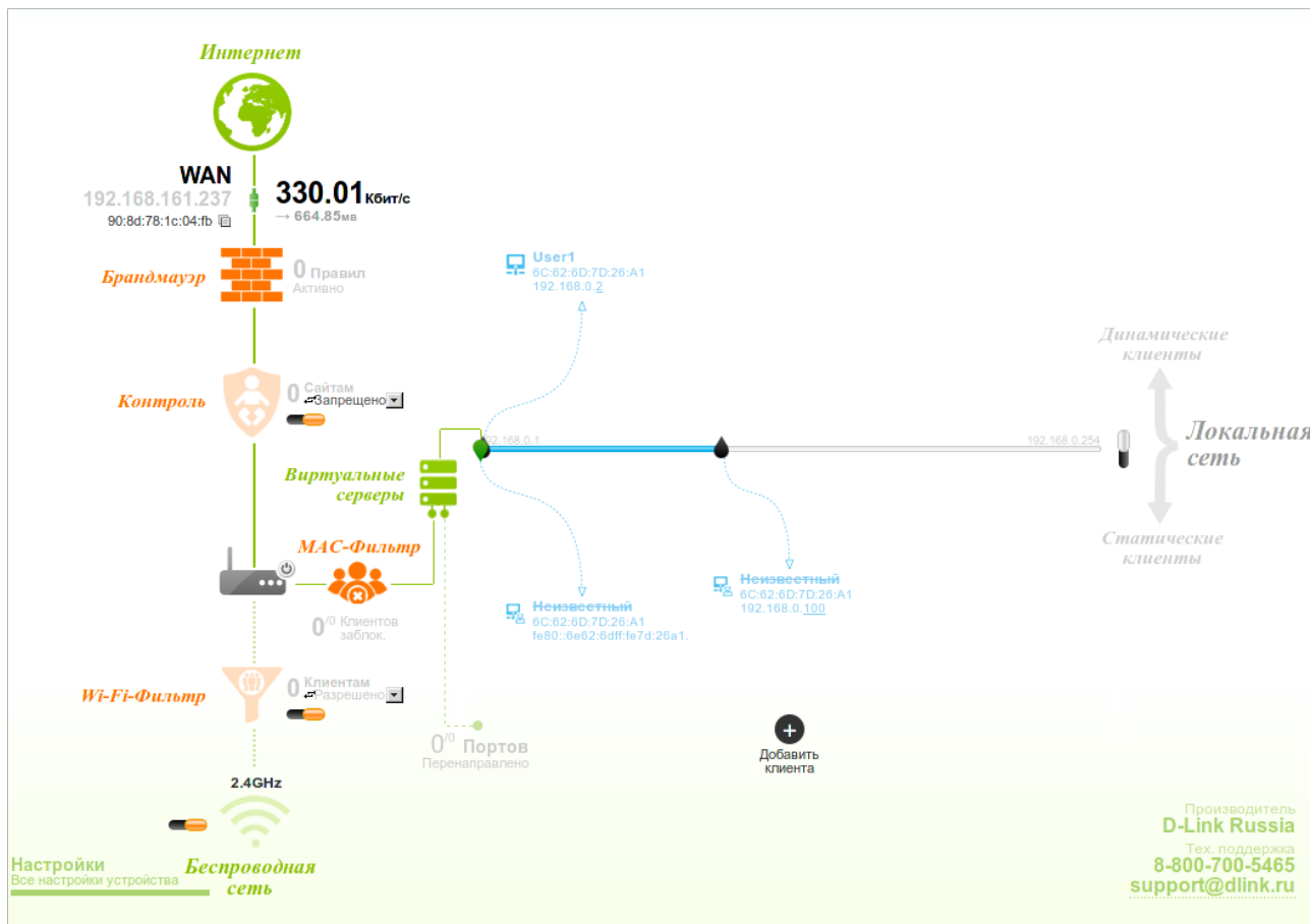
Рисунок 22. Страница Мониторинг .
