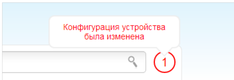
Рисунок 20. Уведомления web-интерфейса.
