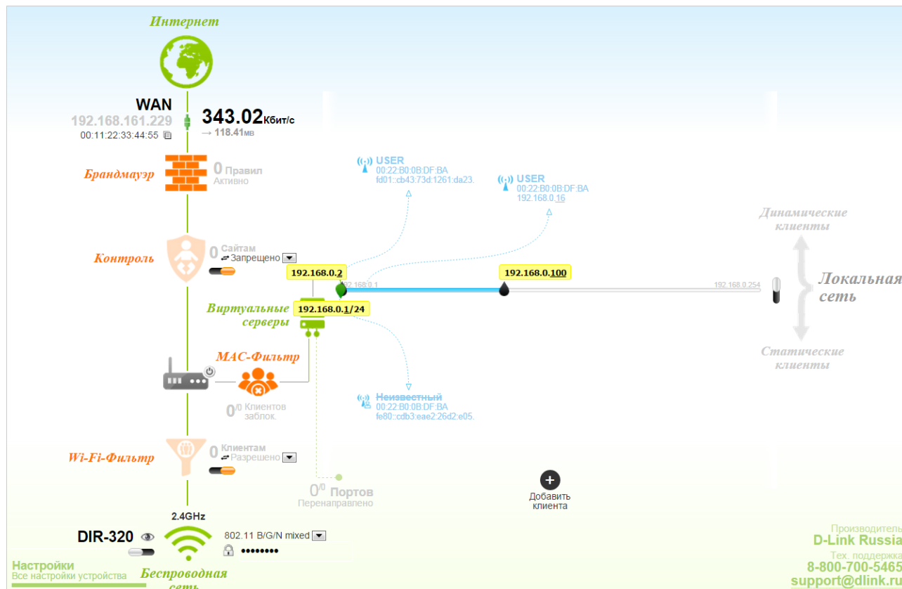
Рисунок 22. Страница Мониторинг .
