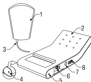
Рис.1 Общий вид ORANGE-2600 1. Модуль приема, 2. Модуль покрытия, 3. Кабель, 4. Индикатор «Тревога», 5. Индикатор «Норма», 6. Разъем SMA, 7. Разъем питания, 8. Разъем USB
