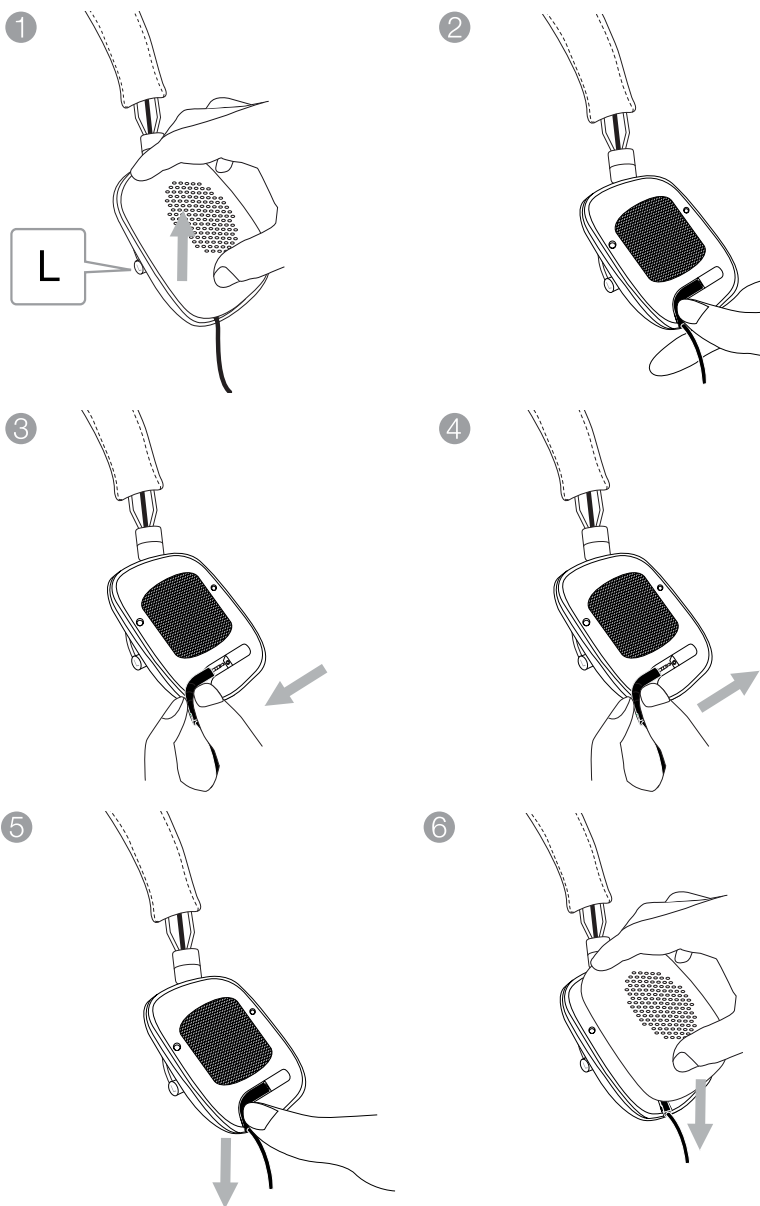
Dibujo 3 Cambio del cable
