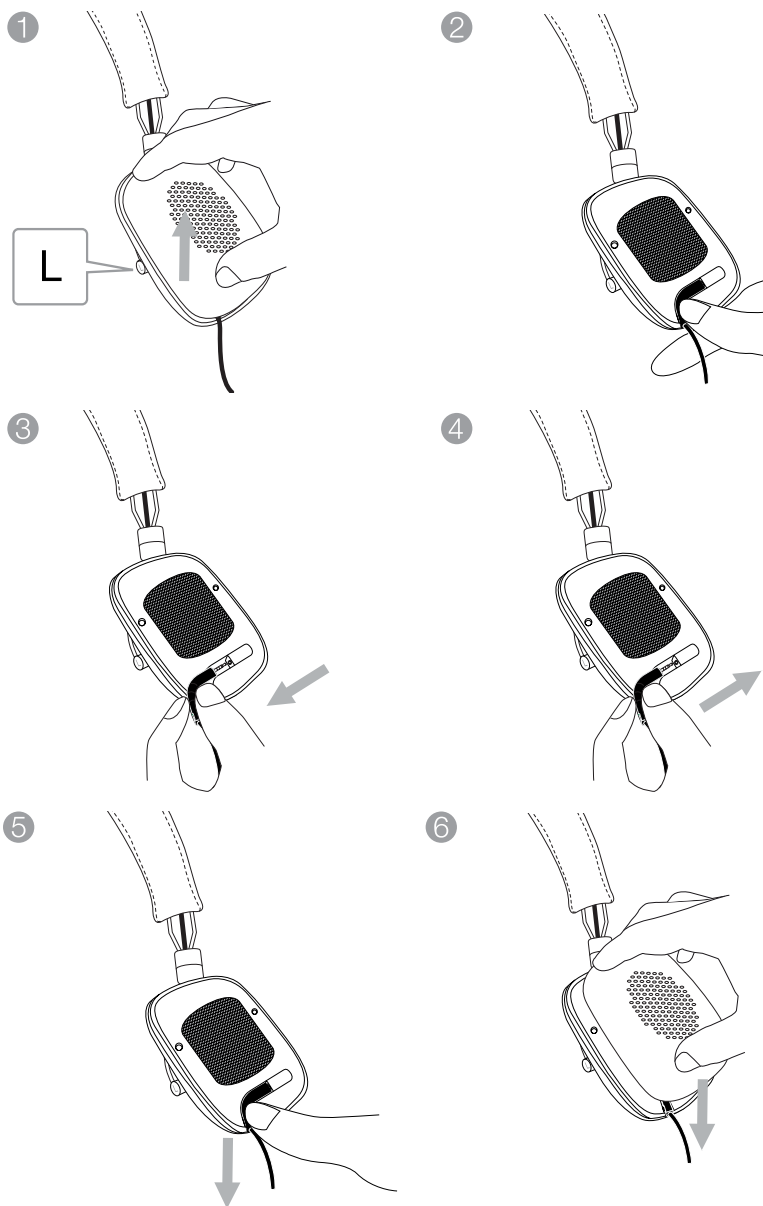
3. Ábra A vezeték cseréje
