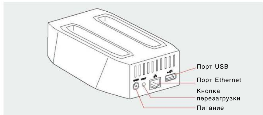
Иллюстрация 2: Устройство GoFlex Net – вид сзади
