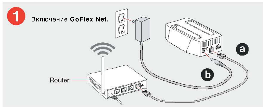
Иллюстрация 3: Подключение Ethernet и источника питания
