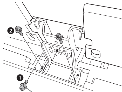
Tornillo de ajuste de ángulo (PSW5 × 10) plateado
