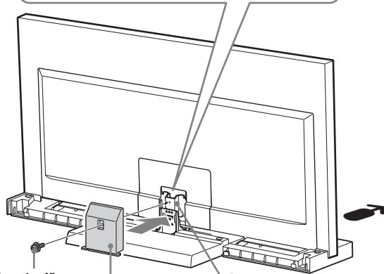
Schraube für Ansatzabdeckung (PSW5 × 16) schwarz Ansatzabdeckung Ansatz
