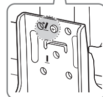
角度調整螺絲 (PSW5 × 10) 銀色
