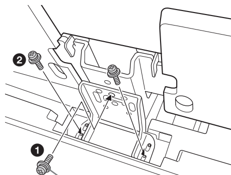
Wkręt do regulacji kąta (PSW5 × 10) srebrny
