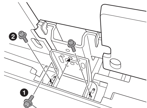
Vite di regolazione inclinazione (PSW5 × 10) argento
