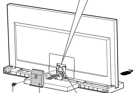
پیچ پوشش گردن (PSW5 × 16) مشکی پوشش گردن گردن
