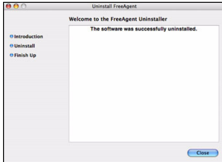
Рис. 32: Удаление завершено
