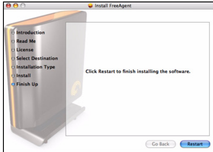
Рис. 12: Перезагрузка
