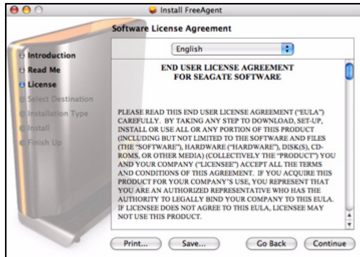
Рис. 6: Лицензионное соглашение
