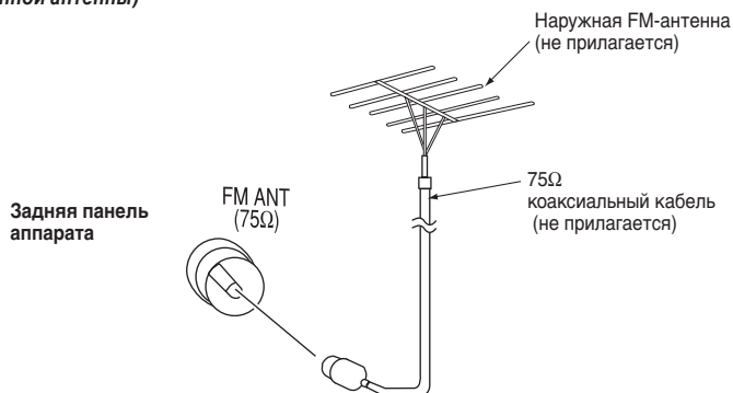
Наружная FM-антенна (Использование телевизионной антенны)
