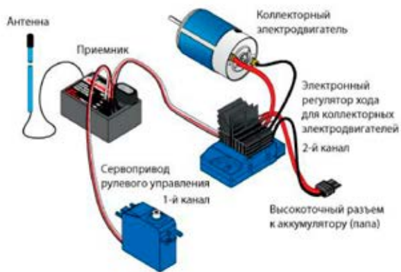
Схема подключения коллекторного электродвигателя
