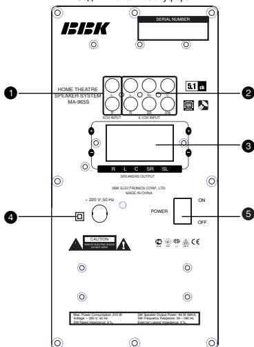
Задняя панель сабвуфера
