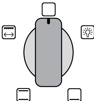
Рис. 4. Переключатель режимов моделей IES 1604 и IES 1624
