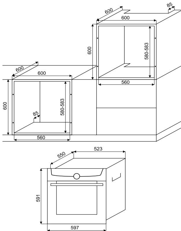
Рис. 8. Схема по встраиванию духового шкафа
