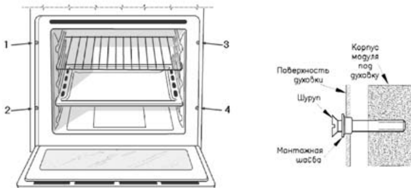
Рис. 9. Крепление духового шкафа к мебели
