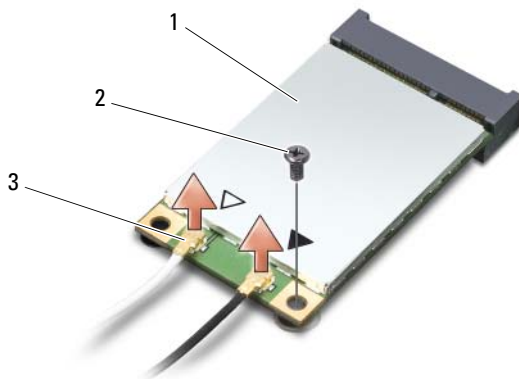
1 плата беспроводной локальной сети 2 винт M2 x 3 мм 3 разъемы антенных кабелей (2)
