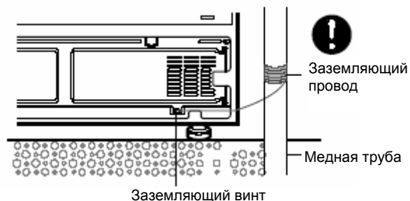
Заземляющий винт
