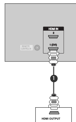
Цифровая приставка
