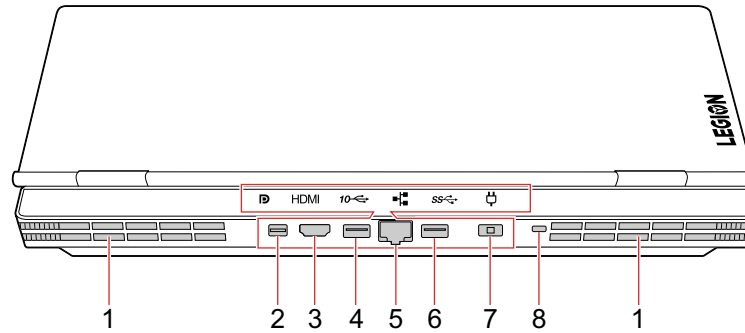
Рис. 5. Lenovo Legion серии Y740–15/17 — вид сзади
