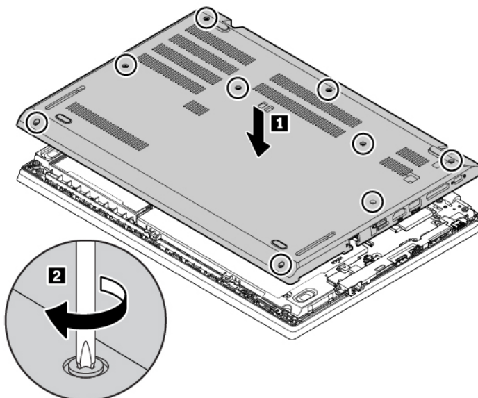
Рис. 6. Установка узла крышки корпуса (для компьютеров ThinkPad L480)
