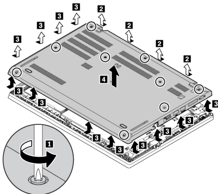
Рис. 4. Снятие узла крышки корпуса (для компьютеров ThinkPad L480)
