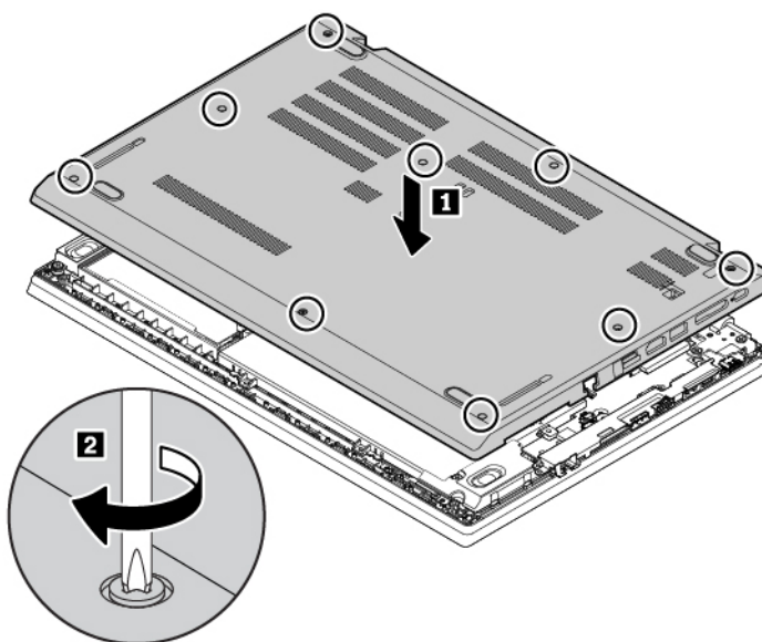
Рис. 7. Установка узла крышки корпуса (для компьютеров ThinkPad L580)
