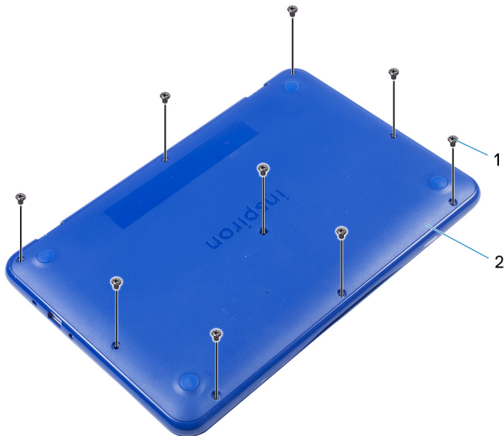
Рисунок 2. Извлечение винтов
