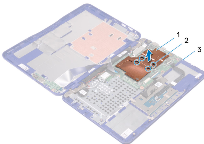
Рисунок 14. Снятие радиатора
