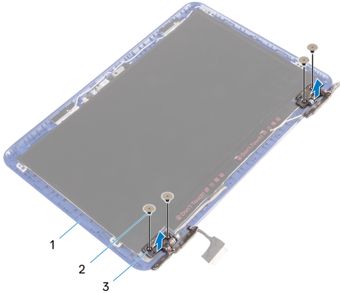
Рисунок 34. Снятие шарниров
