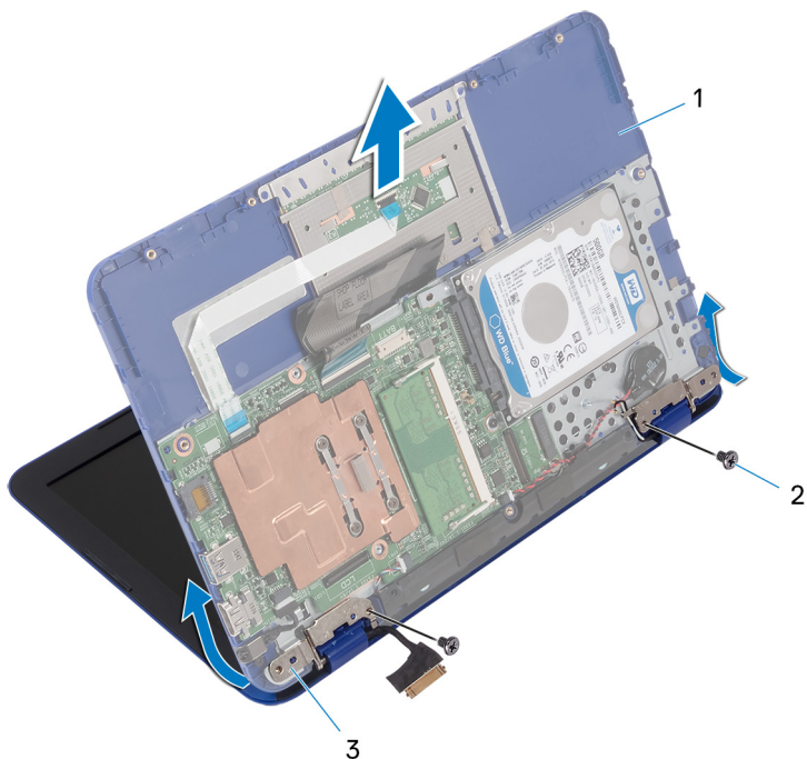
Рисунок 26. Снятие дисплея
