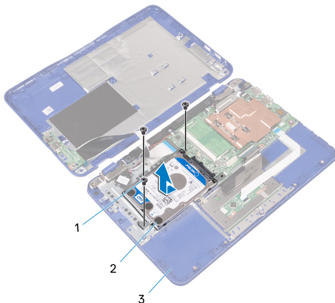
Рисунок 17. Извлечение модуля жесткого диска
