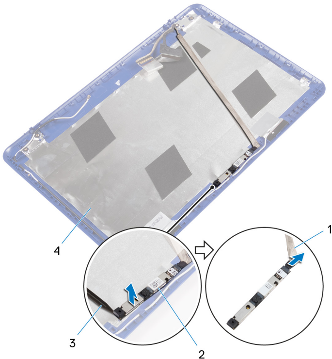
Рисунок 37. Извлечение камеры
