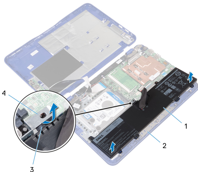
Рисунок 10. Снятие аккумулятора
