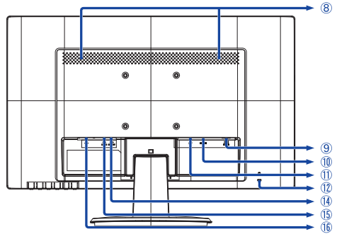
<Вид сзади>
