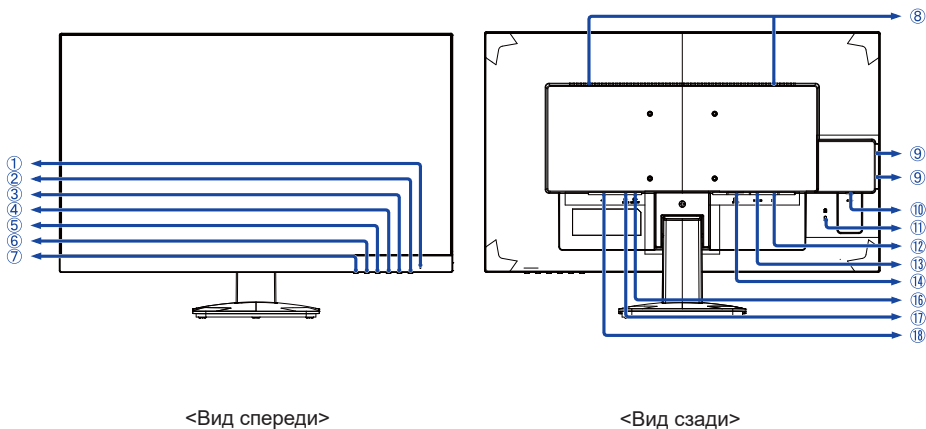
<Вид спереди>
