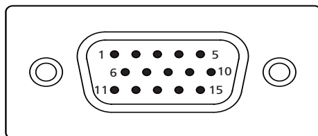
15-контактный сигнальный кабель цветного дисплея
