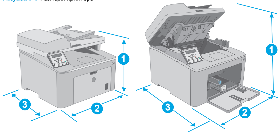
Рисунок 1-1 Размеры принтера
