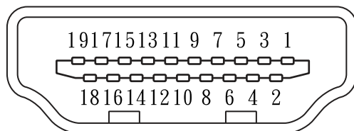
19-контактный сигнальный кабель цветного дисплея
