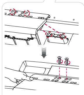
Основание подставки
