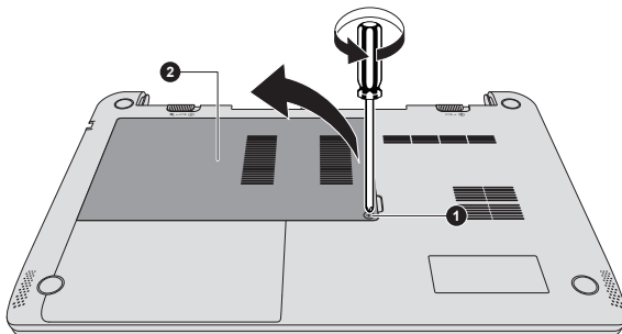
Рисунок 4-7 Снятие крышки отсека модулей памяти
