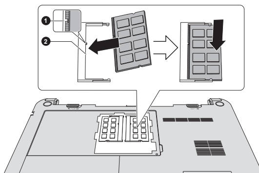
Рисунок 4-8 Установка модуля памяти
