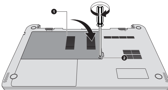
Рисунок 4-9 Установка крышки отсека модулей памяти
