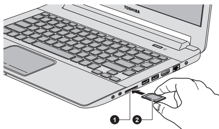
Рисунок 4-12 Установка запоминающего устройства
