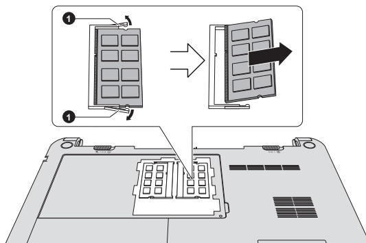
Рисунок 4-10 Удаление модуля памяти
