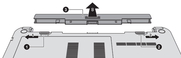
Рисунок 4-6 Высвобождение батарейного источника питания – 1
