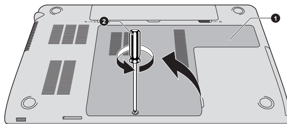
Рисунок 3-13 Снятие крышки отсека модулей памяти
