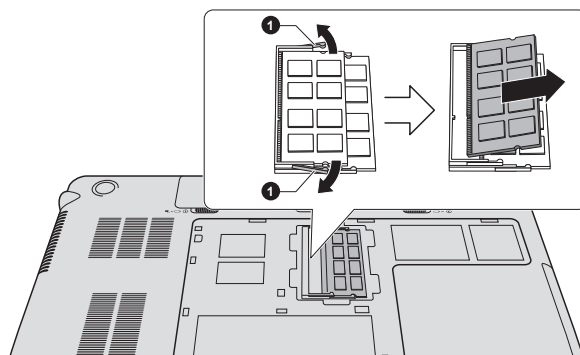
Рисунок 3-16 Удаление модуля памяти
