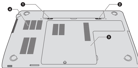
Рисунок 2-5 Вид компьютера снизу
