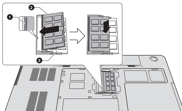
Рисунок 3-14 Установка модуля памяти
