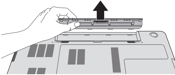
Рисунок 5-2 Высвобождение батарейного источника питания – 2
