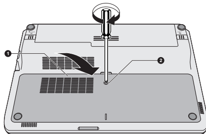
Рисунок 3-12 Установка крышки отсека модулей памяти
