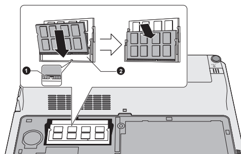
Рисунок 3-11 Установка модуля памяти
