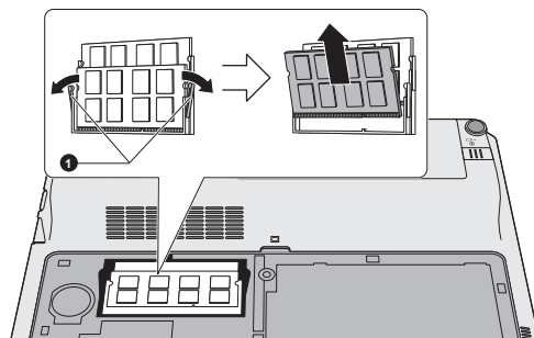
Рисунок 3-13 Удаление модуля памяти
