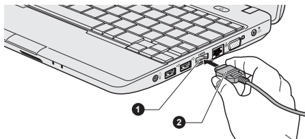
Рисунок 3-15 Подключение к порту выхода HDMI
