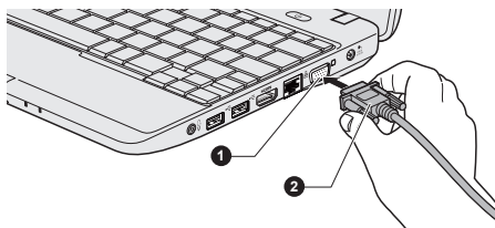
Рисунок 3-14 Подключение кабеля монитора к порту для подключения внешнего монитора RGB
