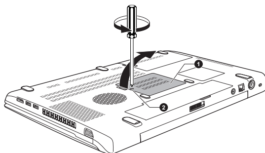
1. Крышка отсека модулей памяти 2. Винт
