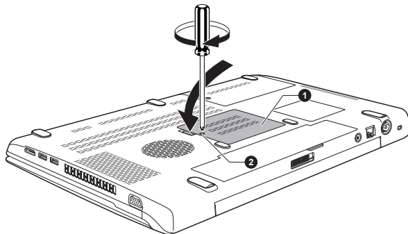
Рисунок 3-13 Установка крышки отсека модулей памяти
