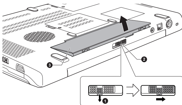
Рисунок 5-1 Высвобождение батарейного источника питания
