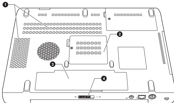
Рисунок 2-5 Вид компьютера снизу
