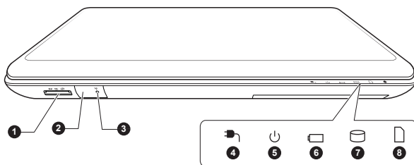
Рисунок 2-1 Вид компьютера спереди с закрытой панелью дисплея
