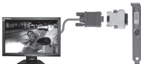
Рис. 2.16. Подключение монитора через переходник DVI/D-Sub
