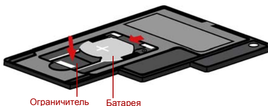
Рисунок 2-15 Удаление батарей
