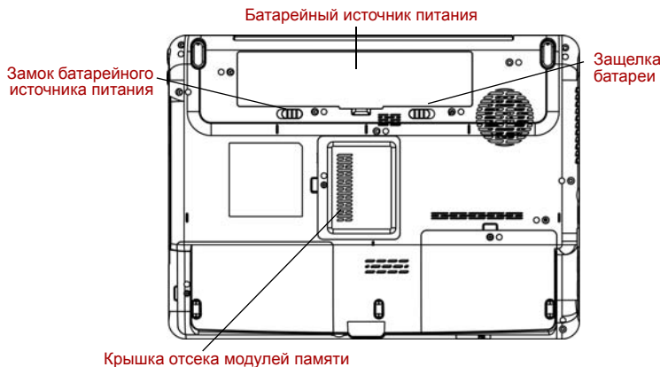
Рисунок 2-5 Вид компьютера снизу
