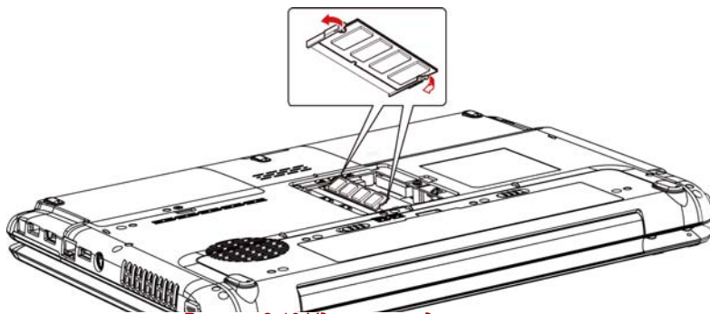
Рисунок 8-10 Удаление модуля памяти
