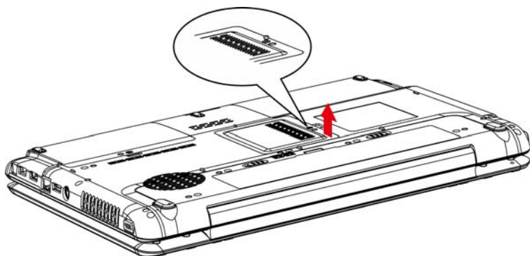
Рисунок 8-7 Снимаем крышку
