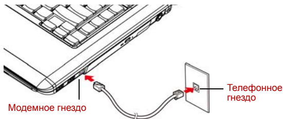
Рисунок 4-14 Подключение встроенного модема
