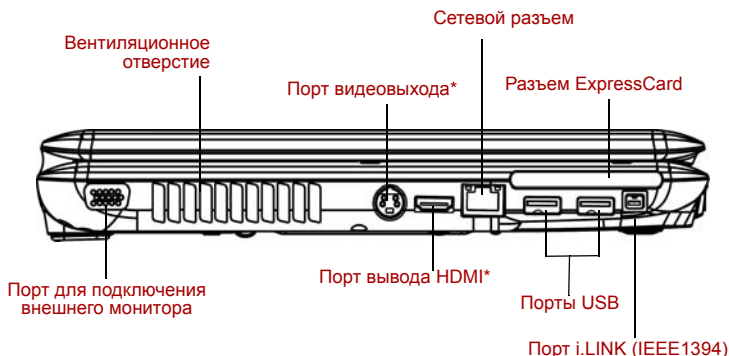
Рисунок 2-2 Вид компьютера слева
