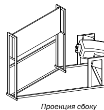
Проекция сбоку
