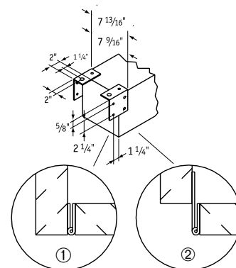
Способ установки экрана: ① стандартной и ② выносной конструкции
