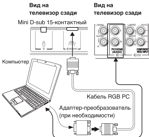
Аудиокабель для соединения ПК и телевизора
