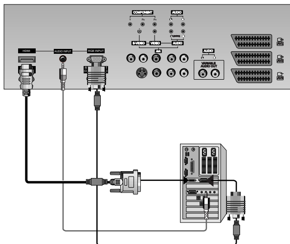
< Задняя панель приемника >
