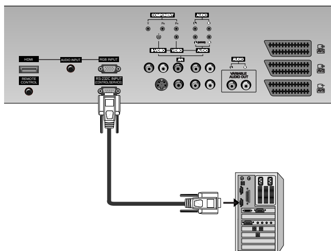
< Задняя панель приемника >
