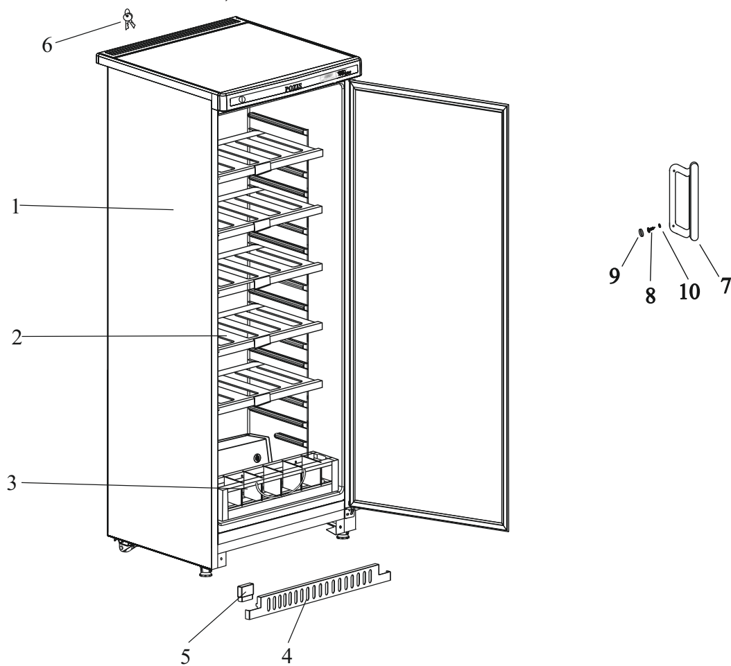
б) ШВ-52 «POZIS»
