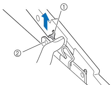
① Задняя монтажная скоба ② Задний штырек
