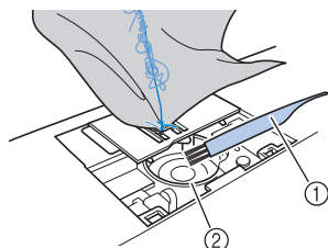
① Щеточка для очистки ② Челнок
