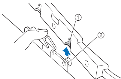
① Передняя монтажная скоба ② Передний штырек
