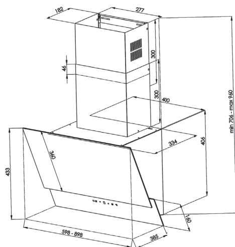
F612 / 912
