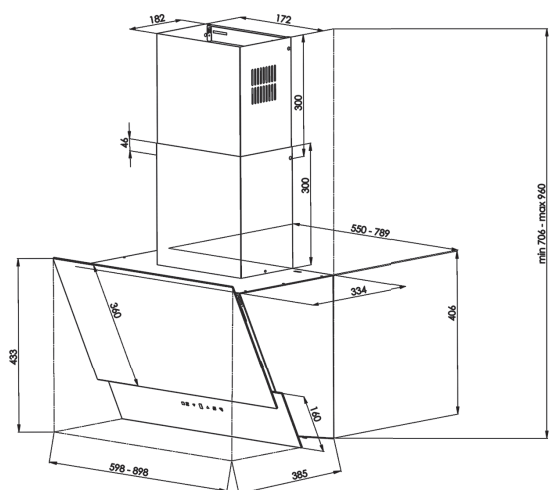
F630 / 930
