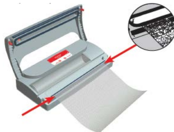
Рисунок 3: Поместите рулон на запечатывающую планку и растяните его до серой силиконовой прокладки, чтобы запечатать (см. стрелки).
