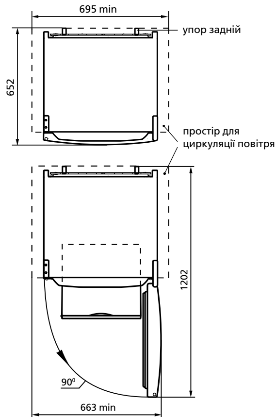
Рисунок 2 – Холодильник (вид зверху)
