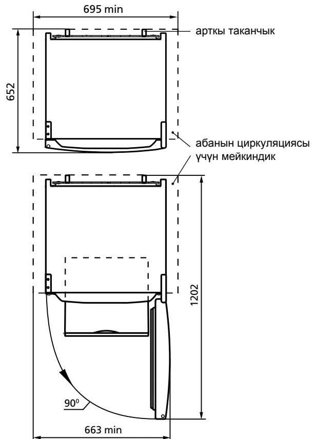
2-сүрөт – Муздаткыч (үстүнөн көрүнүшү)
