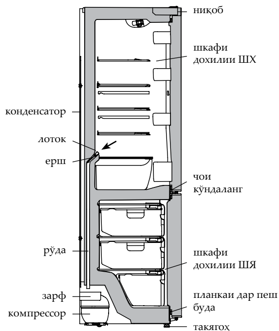
Расми 6 – Нақшаи ректани оби пайдо шуда аз ШХ
