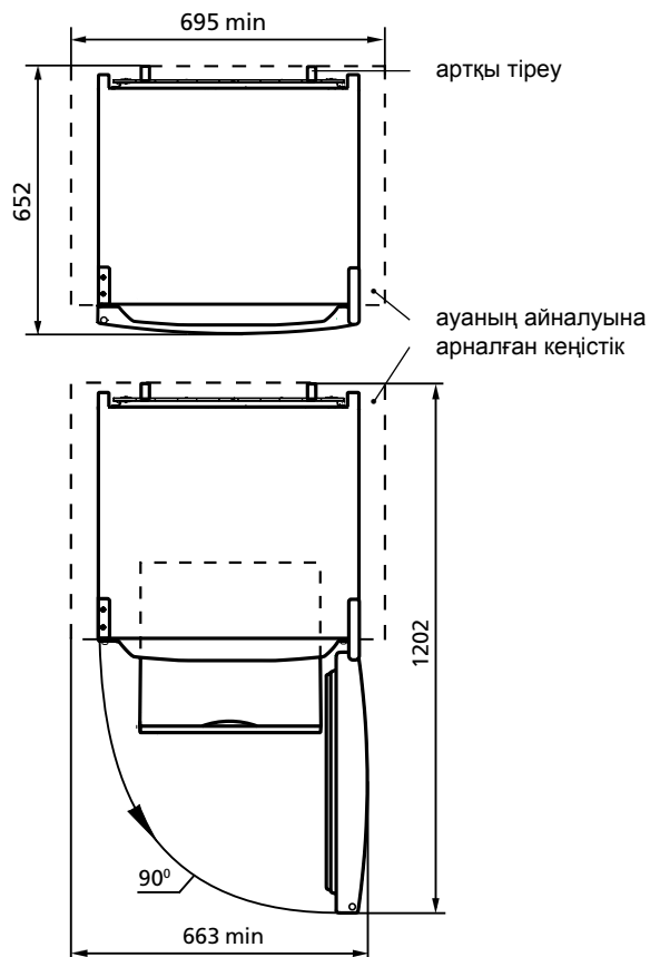
2 сурет – Тоңазытқыш (үстінен көрініс)
