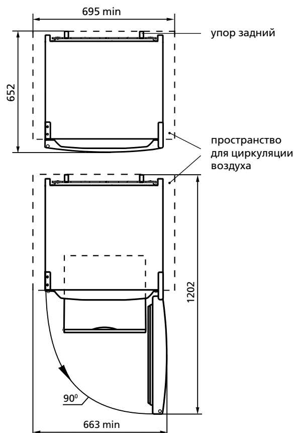
Рисунок 2 – Холодильник (вид сверху)
