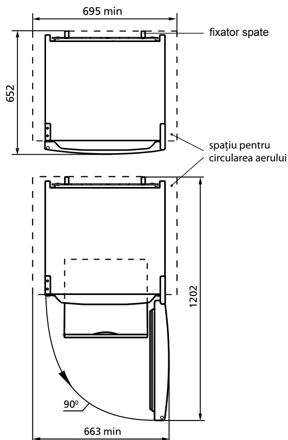
Imagine 2 – Frigider (vedere de sus)
