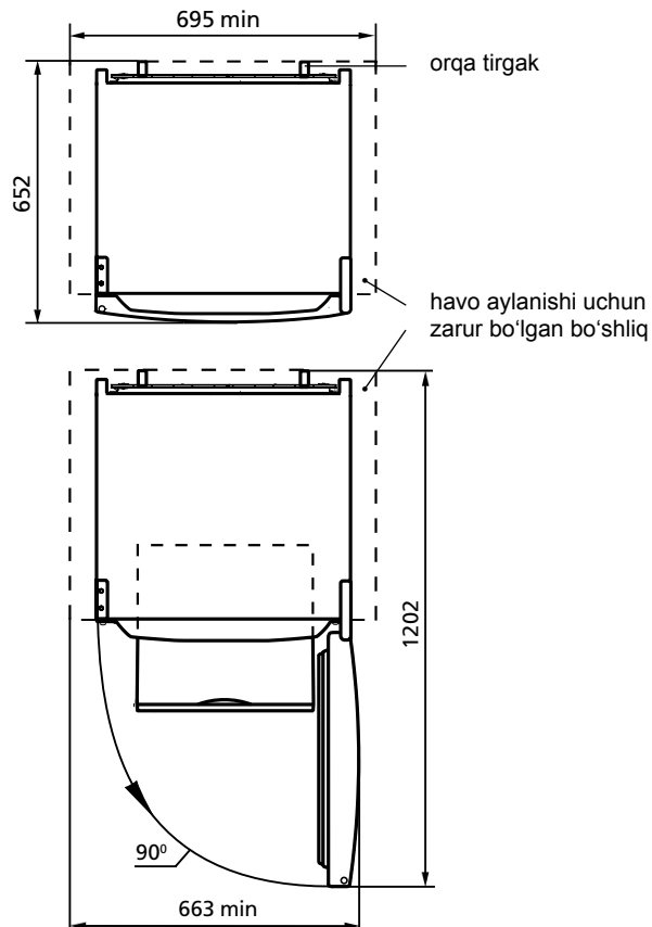
2 Rasm – Sovutgich (ust tomondan ko'rinish)
