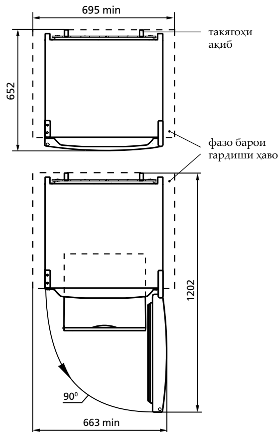
Расми 2 – Яхдон (намуди он аз боло)
