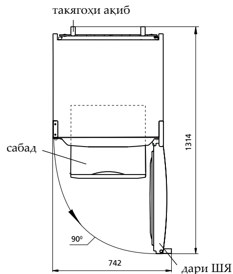
Расми 2 — Яхдон (намуди он аз боло)
