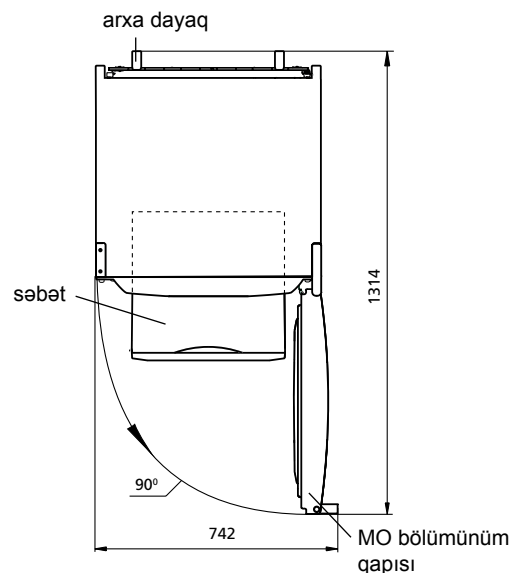
Rəsim 2 — Soyuducu (üstədən görünüşü) bölümünün qapısı
