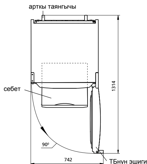
2-сүрөт — Муздаткыч (жогору жагынан көрүнгөн көрүнүшү)
