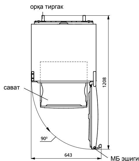
2-расм – Совутқич (уст қисми) кўриниши
