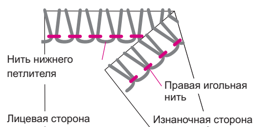
(2) Широкая двухниточная обметочная строчка и Узкая двухниточная обметочная строчка
