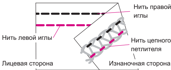
(11) Широкий плоский шов и Узкая плоский шов
