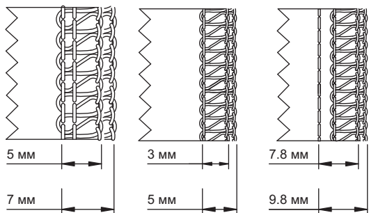
(а) Левая игла (б) Правая игла (с) Цепная игла
