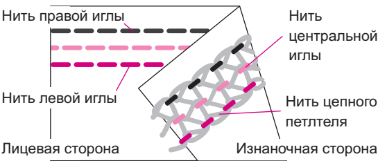
(12) Трехигольный плоский шов
