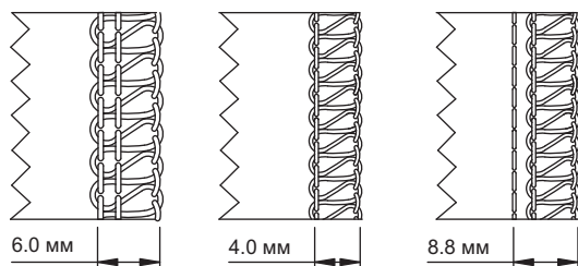
(а) Левая игла (б) Правая игла (с) Цепная игла
