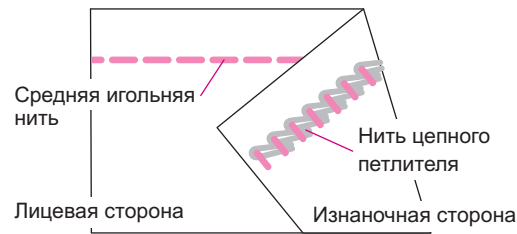
(1) Двойная цепная строчка
