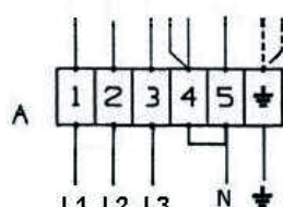
V 400 3N AC 50 Hz
