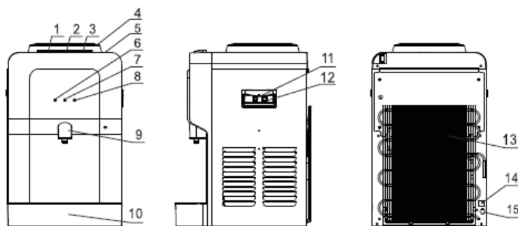
Рис.1. Схема аппарата D910S
