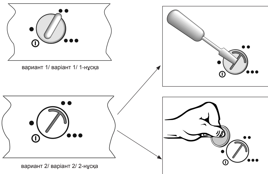
Рисунок Б.3 - Ручка датчика-реле температуры в холодильнике ДХ 416 Рисунок Б.3 - Ручка датчика-реле температуры в холодильнике ДХ 416 Сурет Б.3 - Тетік-реле температурасы тұтқасы тоңазытқыш ДХ 416
