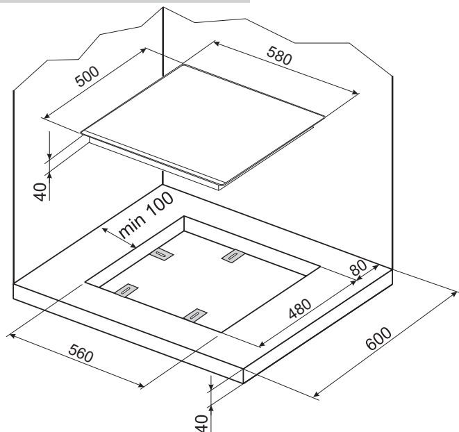
Способ монтажа в мебельном сегменте
