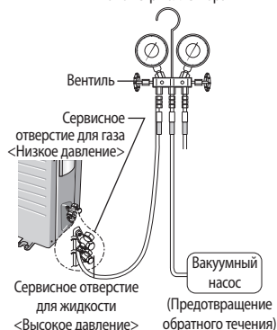
Манометр коллектора
