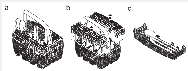
Размещение крышки корзины для столовых приборов (в верхней корзине)
