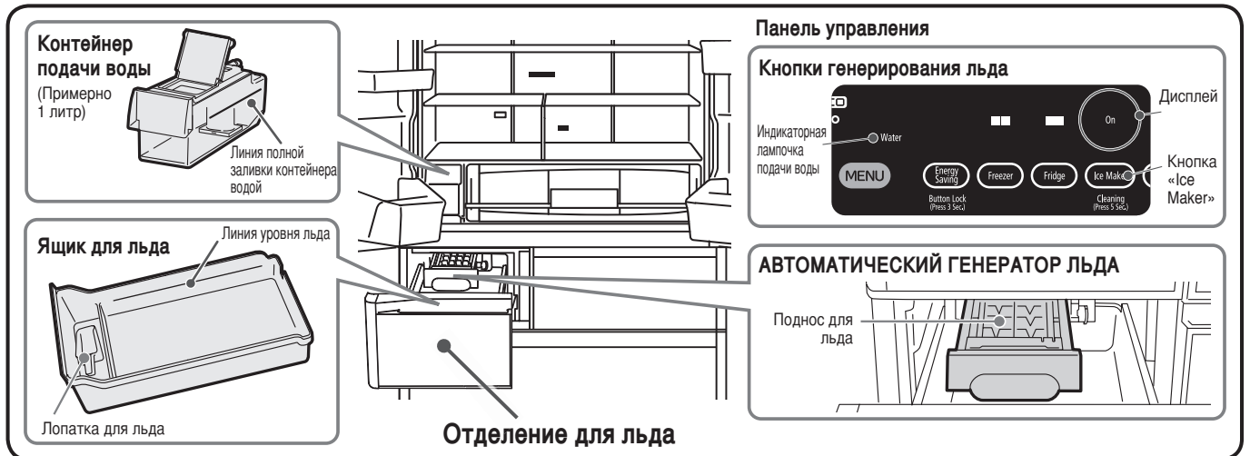
Отделение Для Льда
